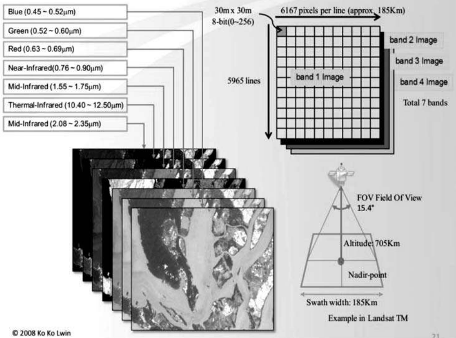
Fig. 3.3 : Bands
